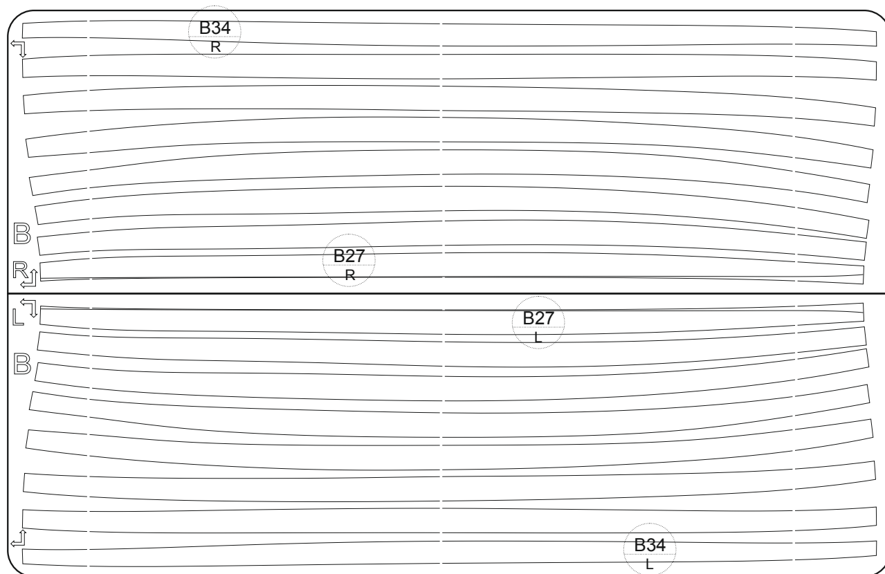
Пластина N / Plate N
