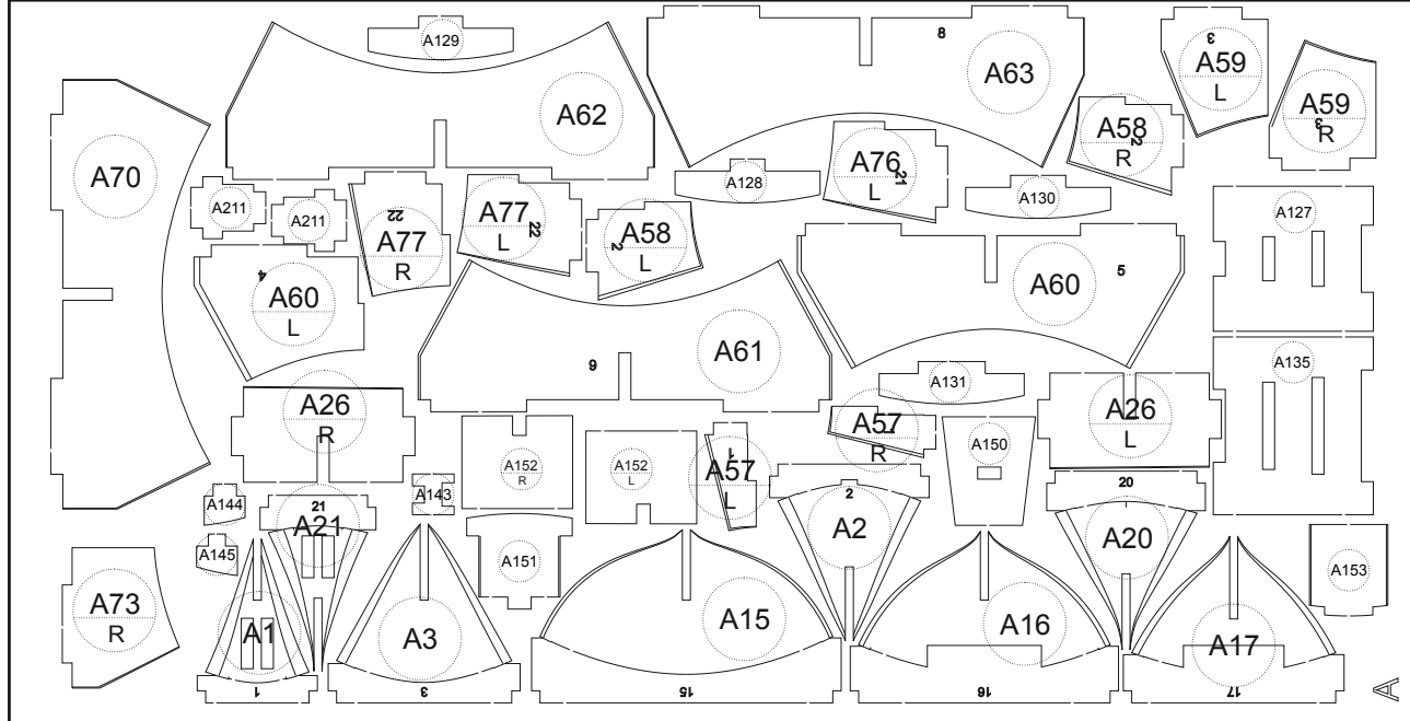
Пластина А (часть 2) Plate A (part 2)
