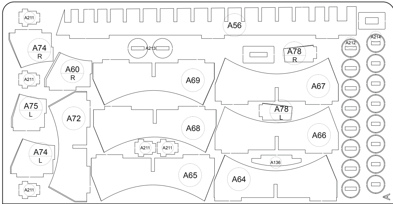
Пластина А (часть 1) Plate A (part 1)
