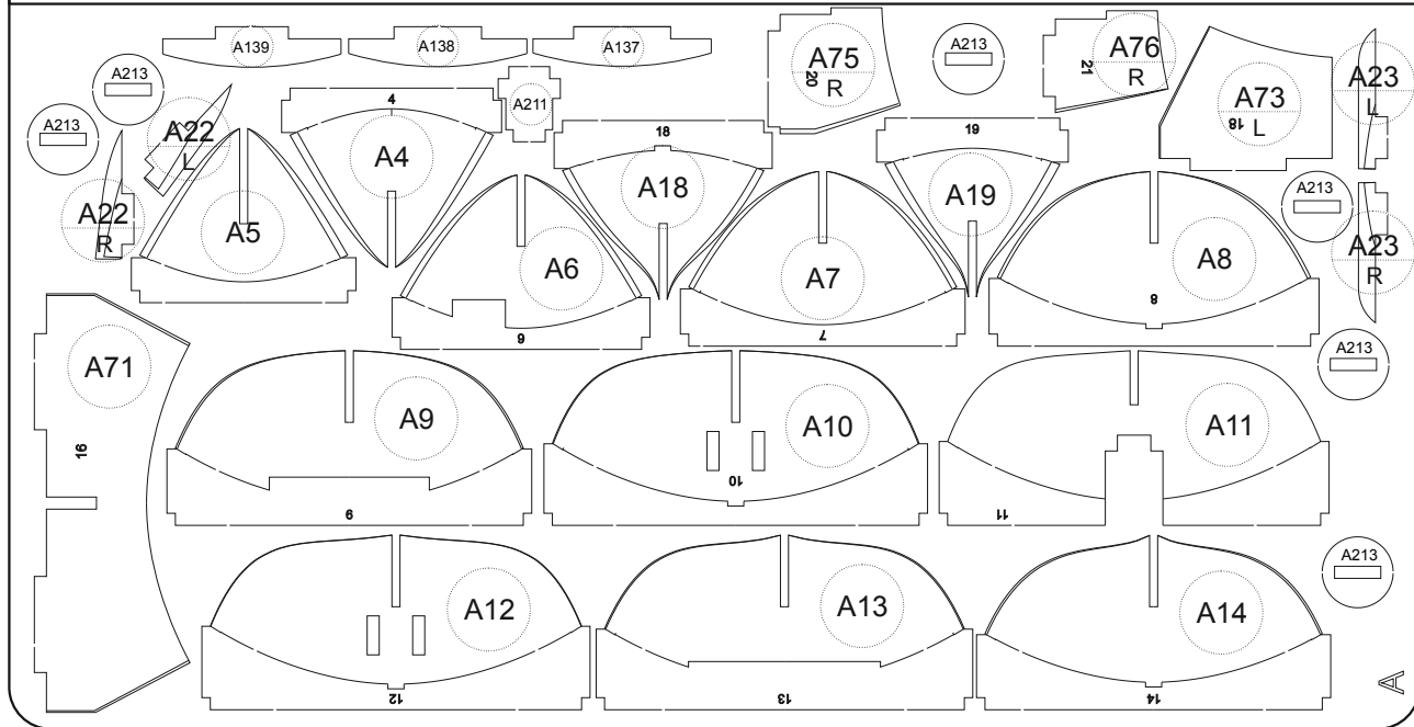
Пластина А (часть 3) Plate A (part 3)
