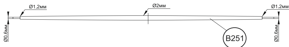
Реек грота-топселя M1:1
