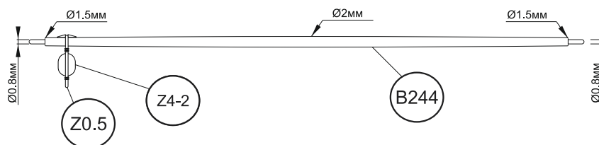
Стаксель-гик M1:1
