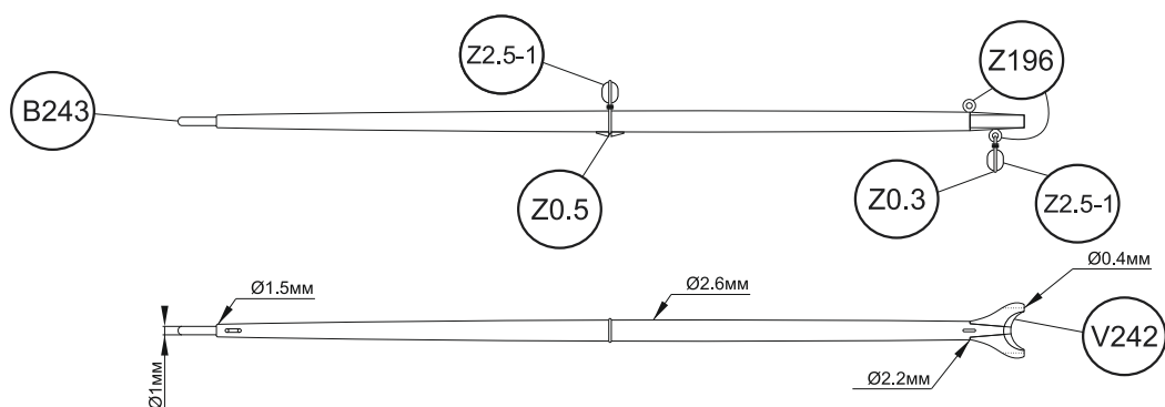
Грота-гафель M1:1
