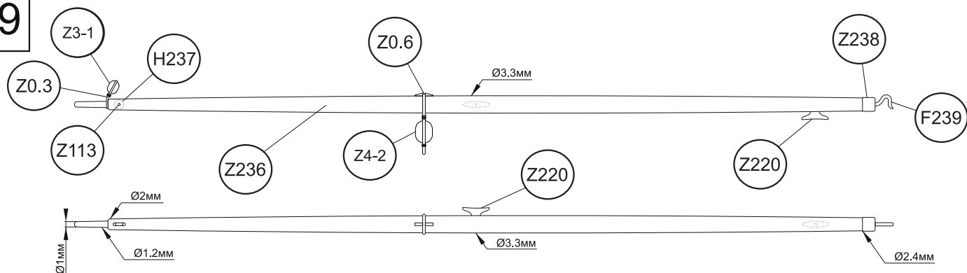
Грота-гик M1:1
