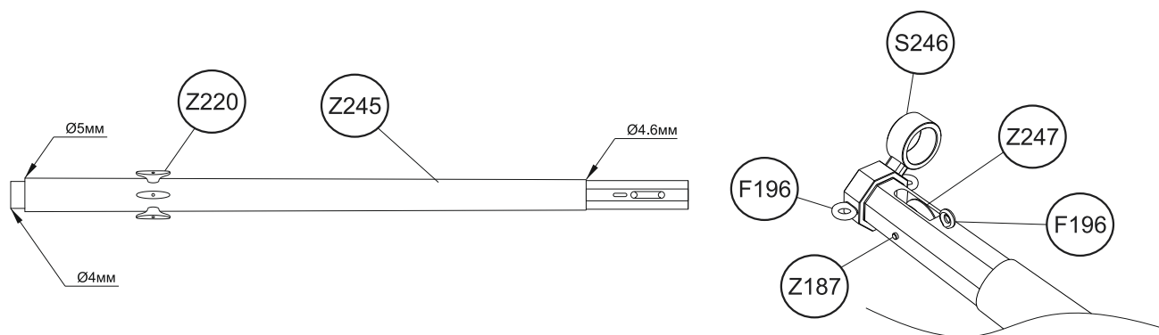
Бушприт M1:1
