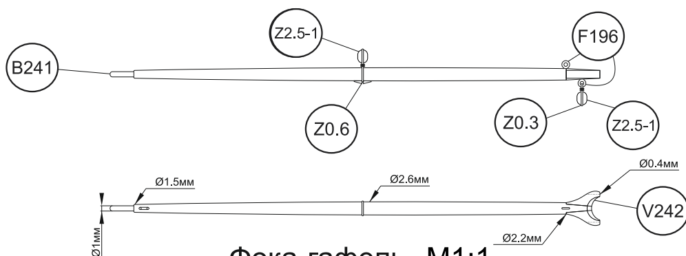
Фока-гафель M1:1
