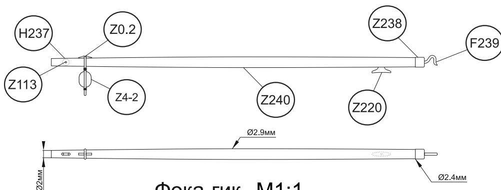
Фока-гик M1:1
