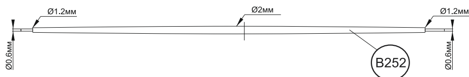
Реек фока-топселя M1:1
