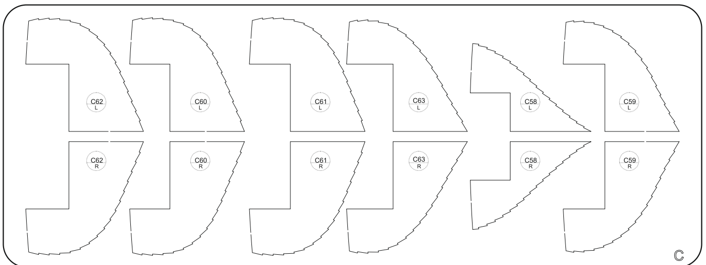
Пластина С (часть2) / Plate C (part2)
