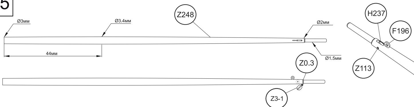
Утлегарь M1:1
