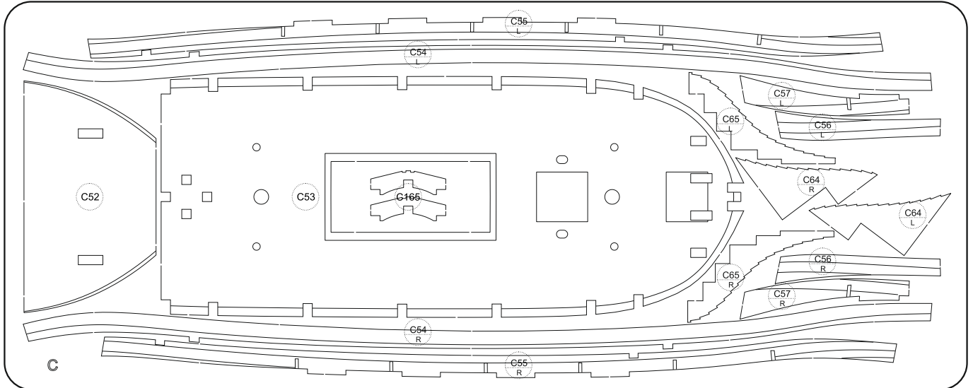
Пластина С (часть2) / Plate C (part2)
